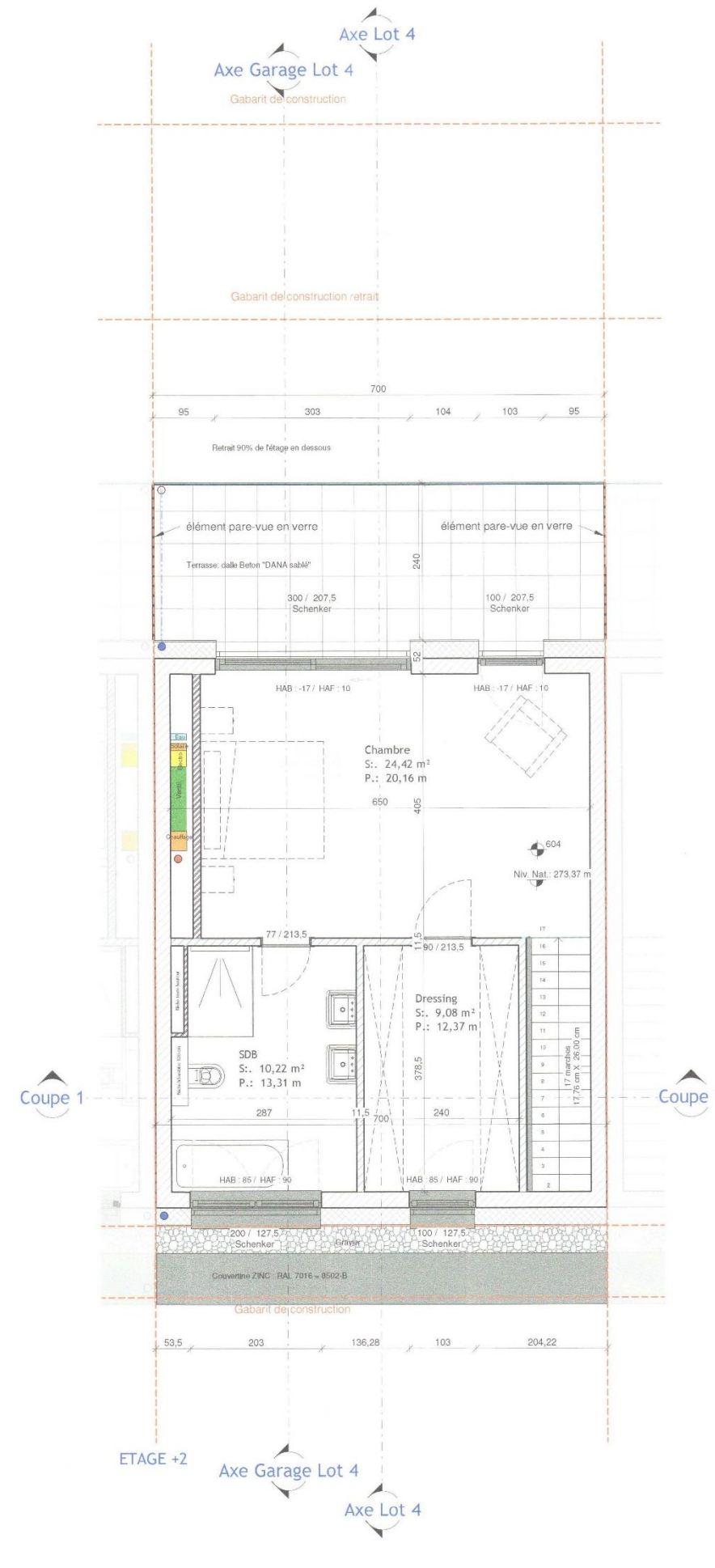
Etage 2
