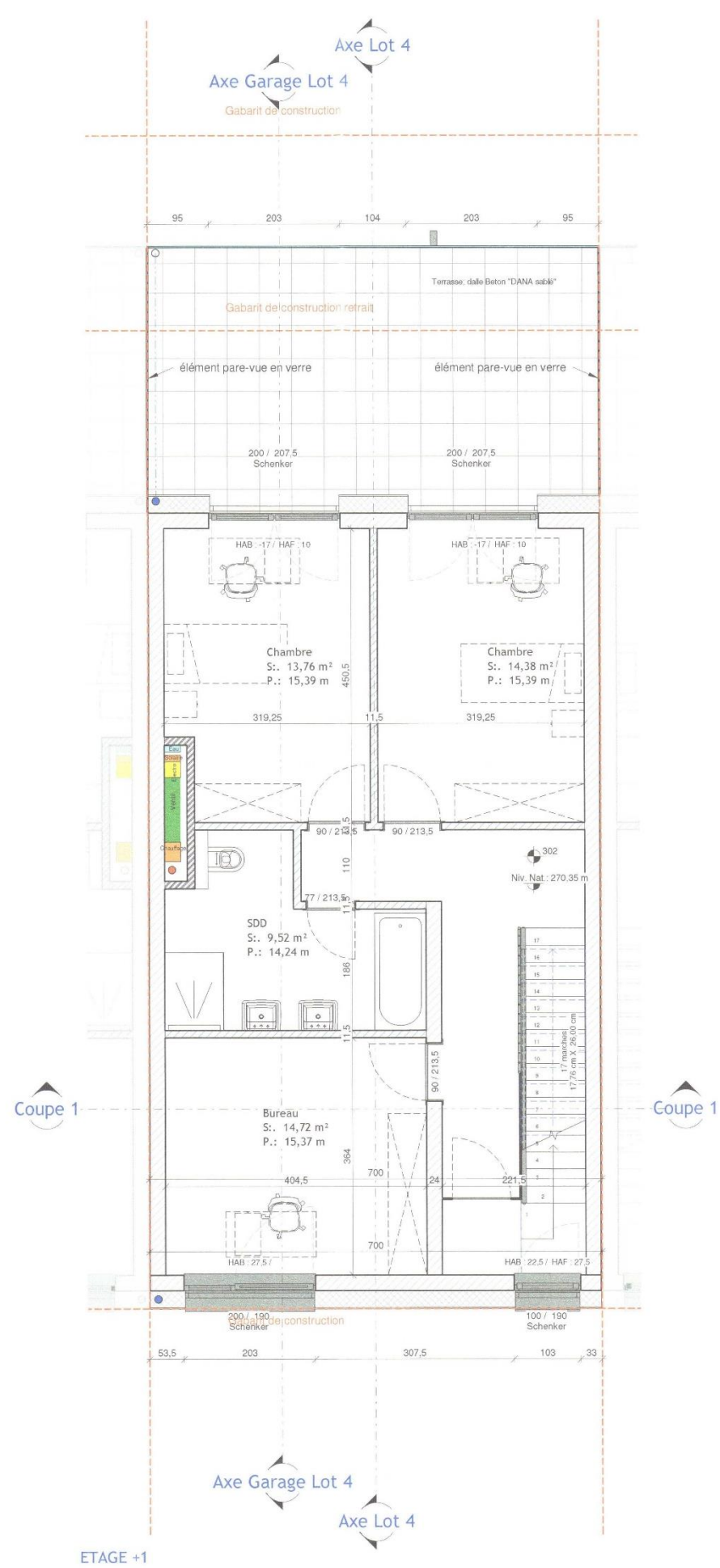
Etage 1
