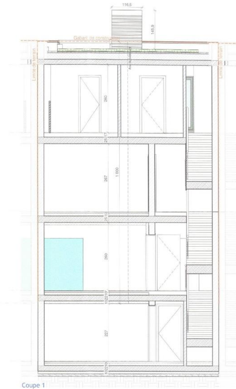
Coupe 1
