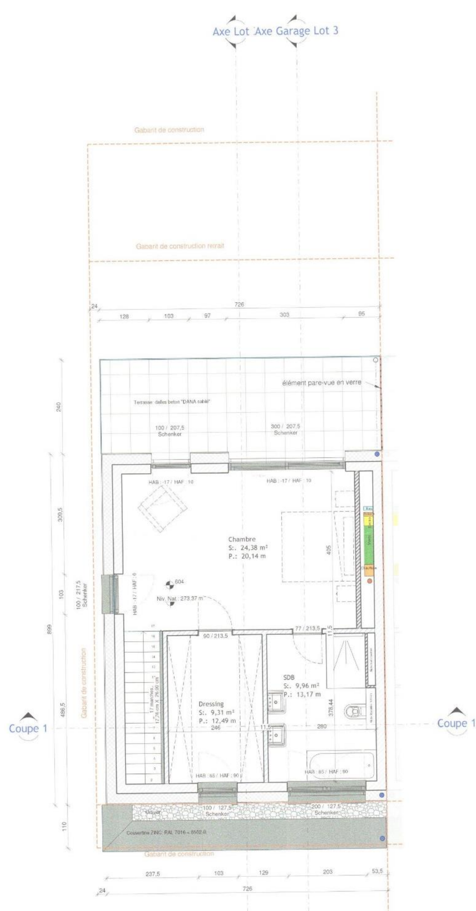
Etage 2
