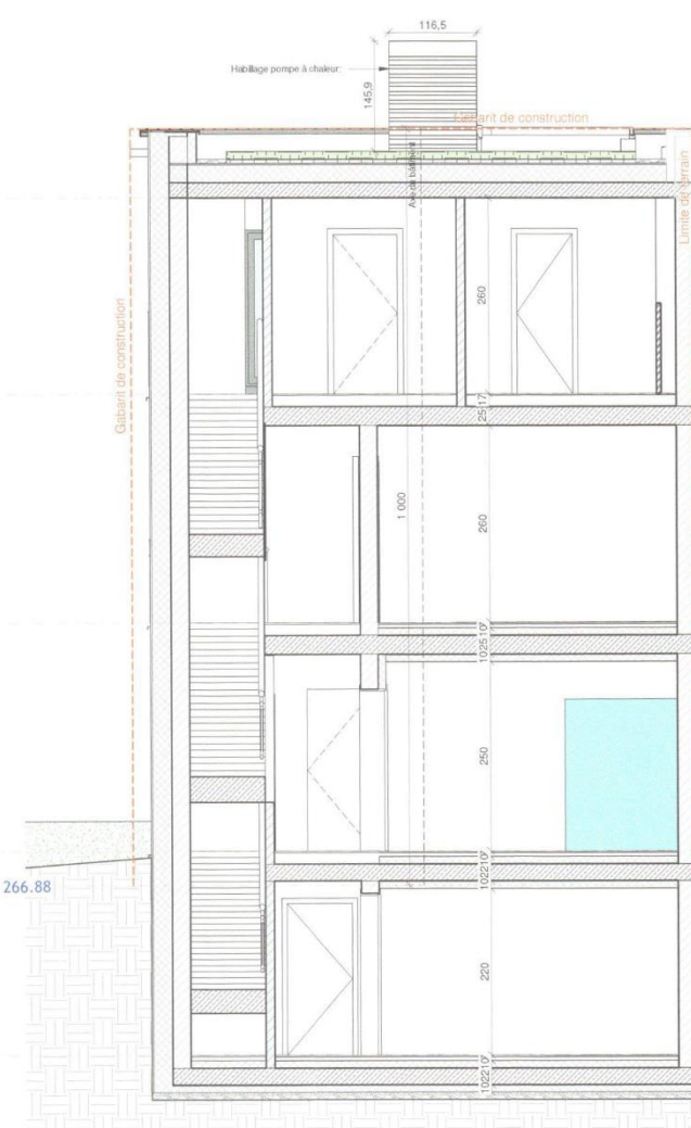
Coupe 1
